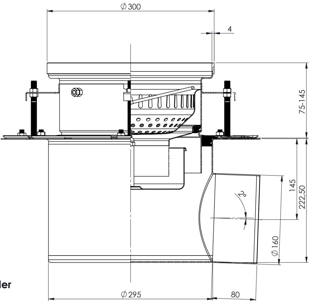
□ Płyta szczelna Tight cover H=25/8mm M125
