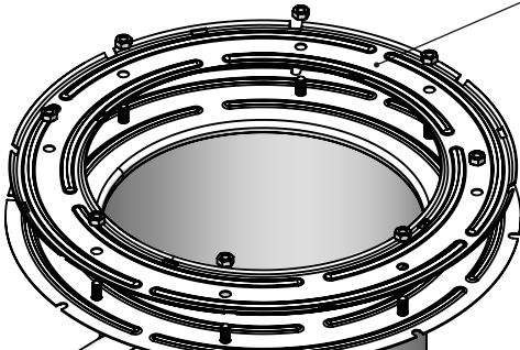
Kołnierz dociskowy Clamping flange
