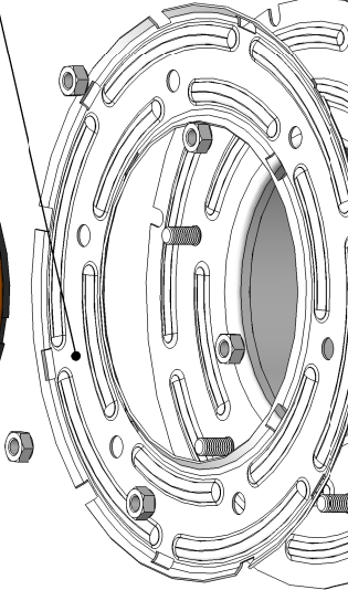
Kołnierz dociskowy Clamping flange
