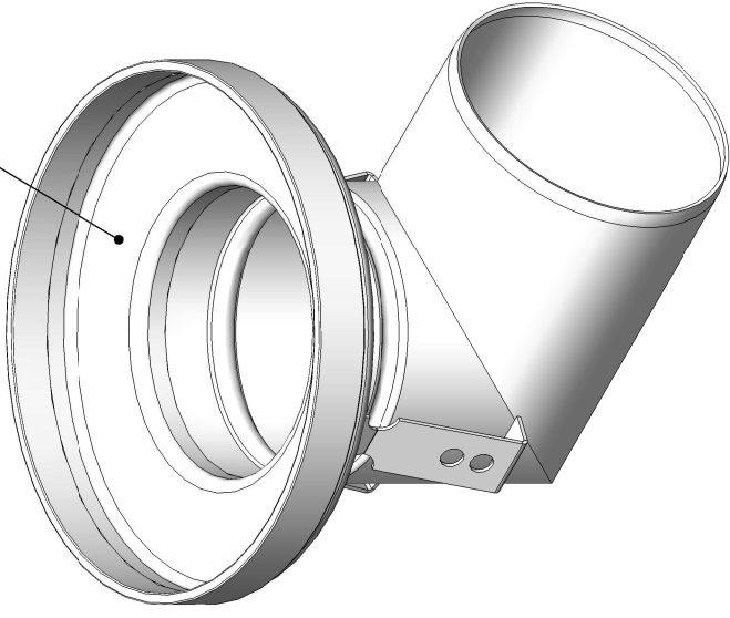
Korpus Body
