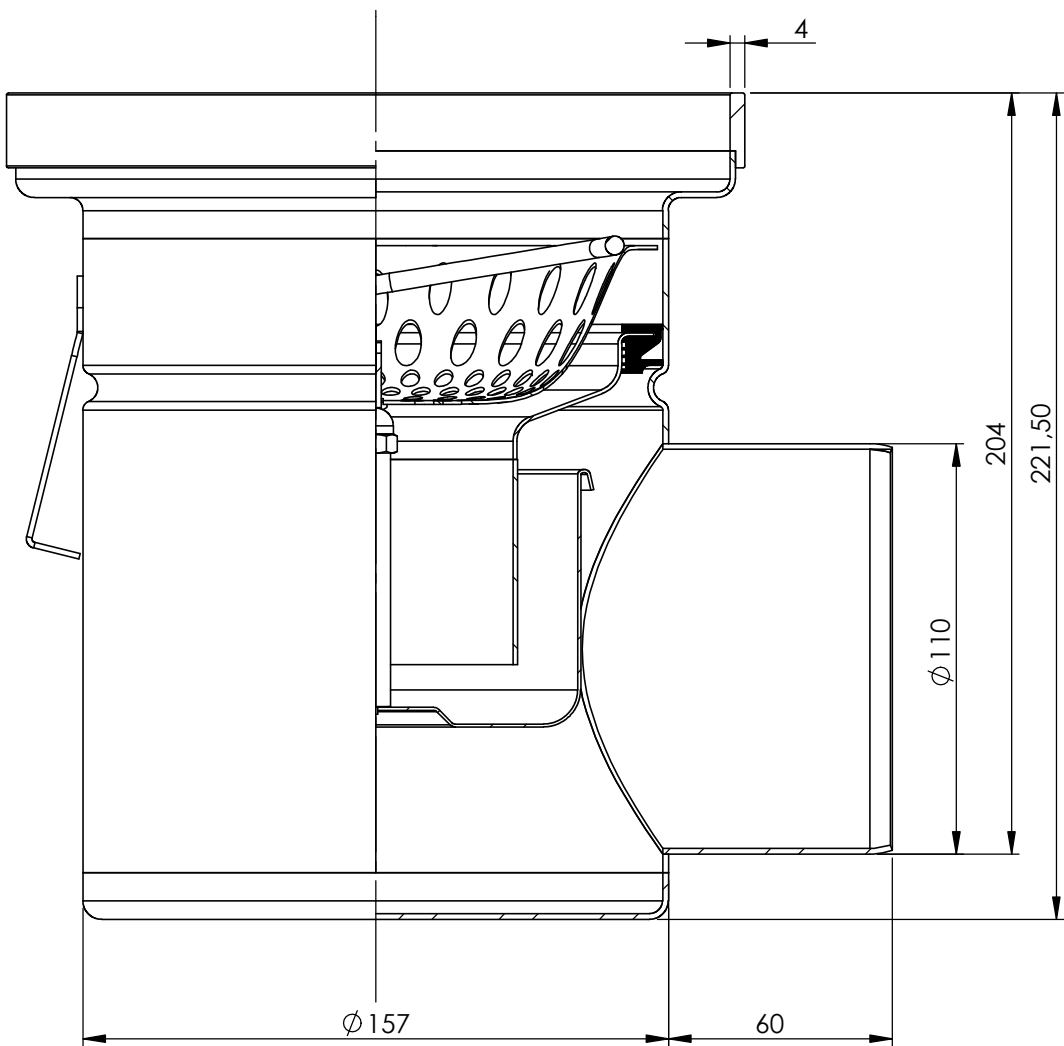
PRZĘKRÓJ A-A
